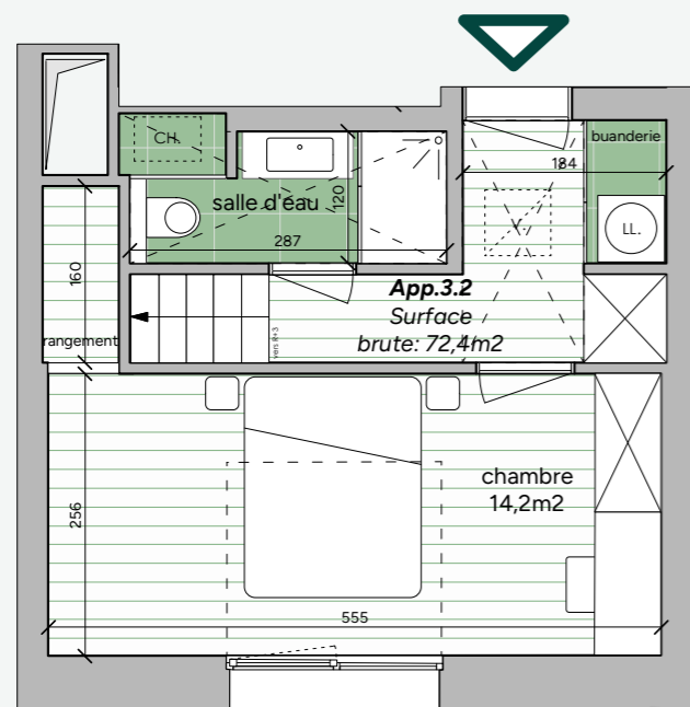
ÉTAGE +2
